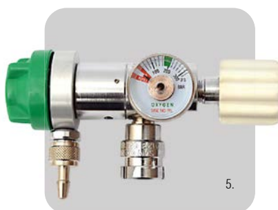
5. Reductor de presión de Pistón con regulación de caudal por puntos. La boquilla es orientable 360° facilitando la introducción de la cánula nasal y/o máscara.
